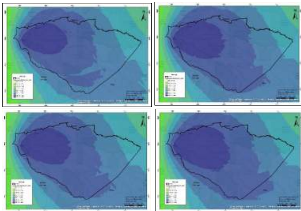
Figura 6. Precipitaciones para el período 2041-2070
