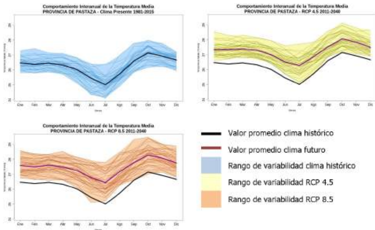
Figura 25: Comportamiento de la temperatura media en Pastaza (clima histórico, emisiones medias – RCP 4.5 y emisiones altas – RCP 8.5).
