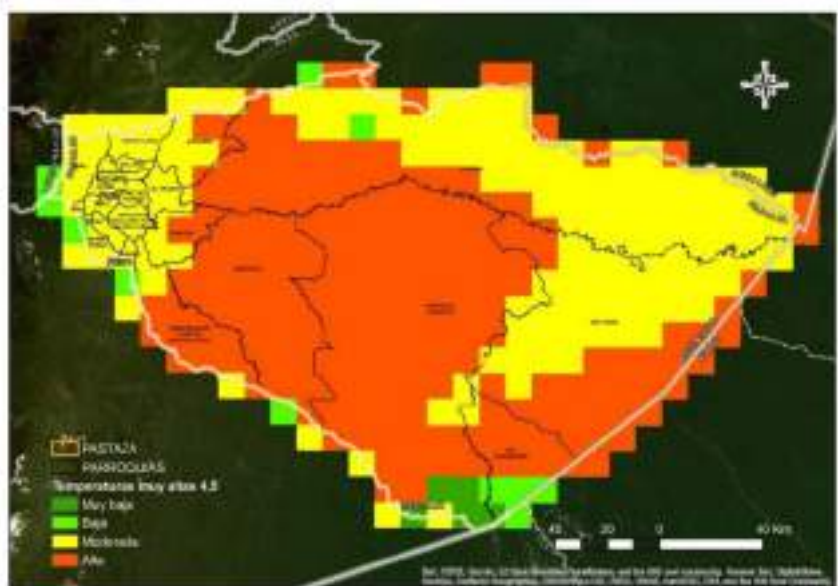
Figura 41. Temperaturas muy altas escenario 4,5
