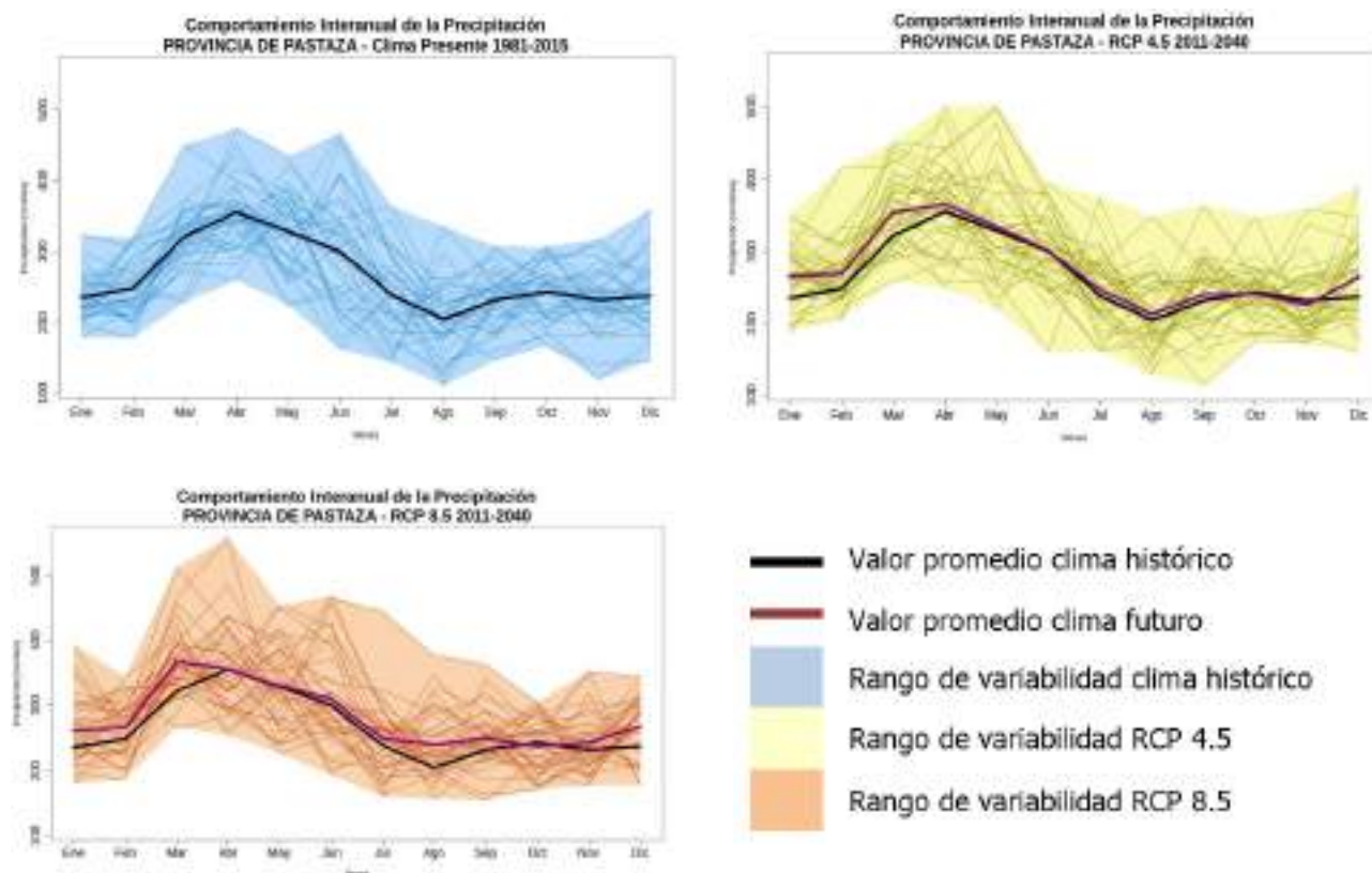
Figura 24: Comportamiento de las precipitaciones en Pastaza (clima histórico, emisiones medias – RCP 4.5 y emisiones altas - RCP 8.5)
